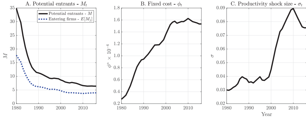
Figure 4: Parameter estimates
